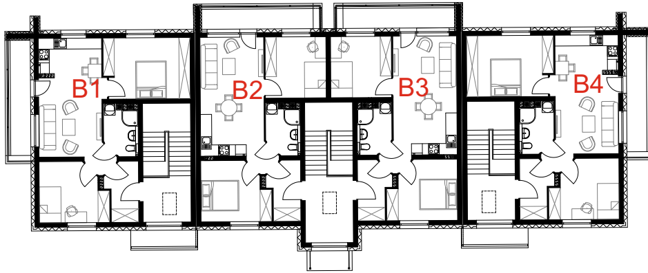
SEGMENT „ B”
